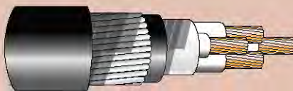
SWA : Galvanized Steel Wire Armoured (Giáp sợi thép mạ kẽm)
